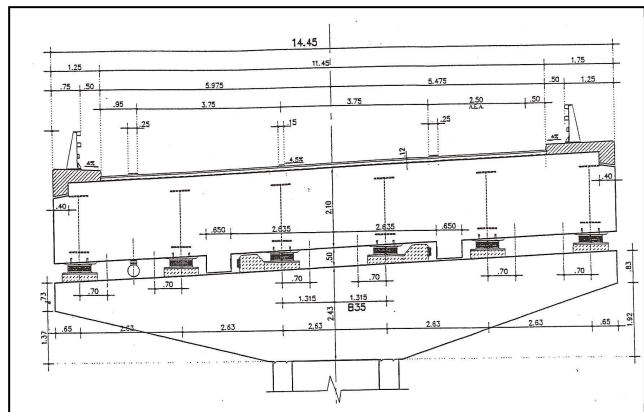
Σχ. 1 Τυπική Διατομή της Γέφυρας
