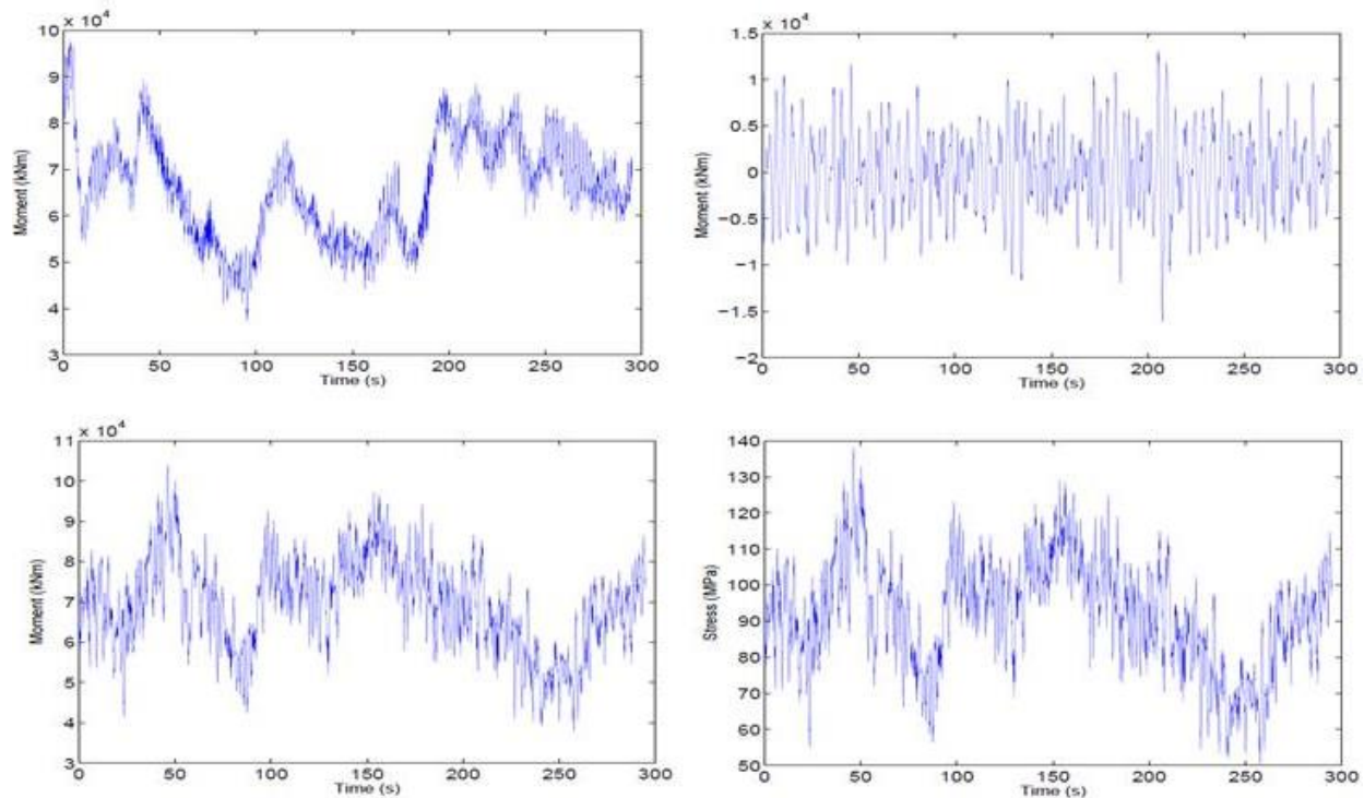
Σχ. 2: α) Χρονοσειρά ροπής λόγω ανέμου, β) Χρονοσειρά ροπής λόγω κυματισμών, γ) Χρονοσειρά συνολικής ροπής στη θεμελίωση, δ) Χρονοσειρά ορθών τάσεων στη θεμελίωση
