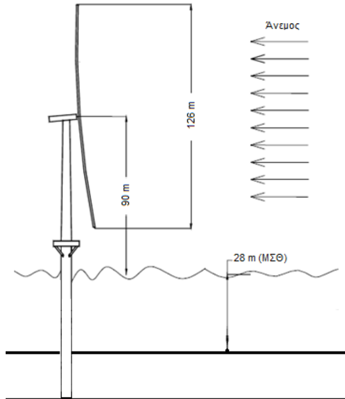
Σχ. 1: Σκαρίφημα κατασκευής και χαρακτηριστικές διαστάσεις
