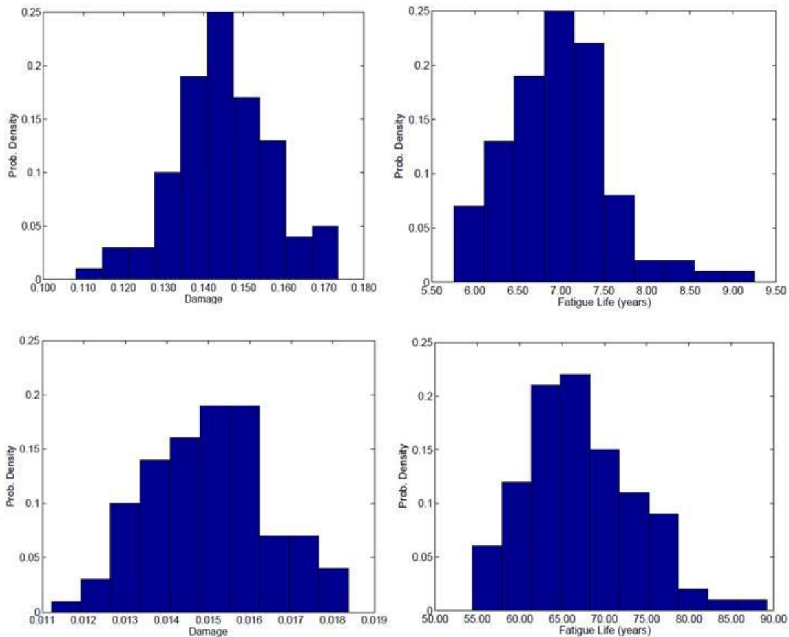
Σχ. 3: (α, β) Κατανομή ετήσιας φθοράς και προβλεπόμενης διάρκειας ζωής λόγω κόπωσης για κατηγορία λεπτομέρειας 40 (γ, δ) Κατανομή ετήσιας φθοράς και προβλεπόμενης διάρκειας ζωής λόγω κόπωσης για κατηγορία 71
