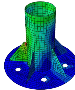
Σχ. 2(β). Προσομοίωμα Π.Σ. της έδρασης των ορθοστατών .
