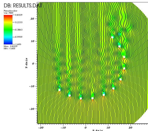
Σχ. 1 (β). Αποτελέσματα ανάλυσης για γωνία προσβολής 45^\circ .
